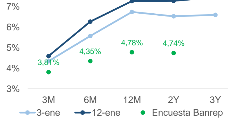
IBR implícita
